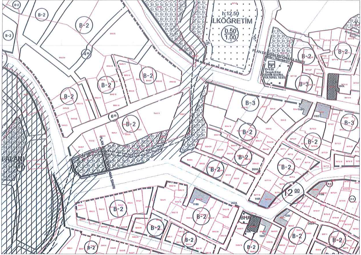
Resim 6. Öneri 1/1000 ölçekli Uygulama İmar Planı Değişikliği
