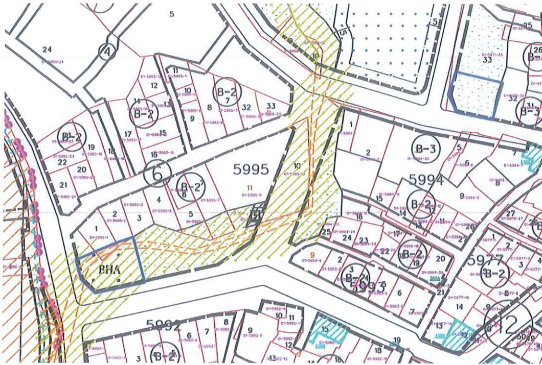
Resim 4.Onaylı 1/1000 ölçekli Uygulama İmar Plan
