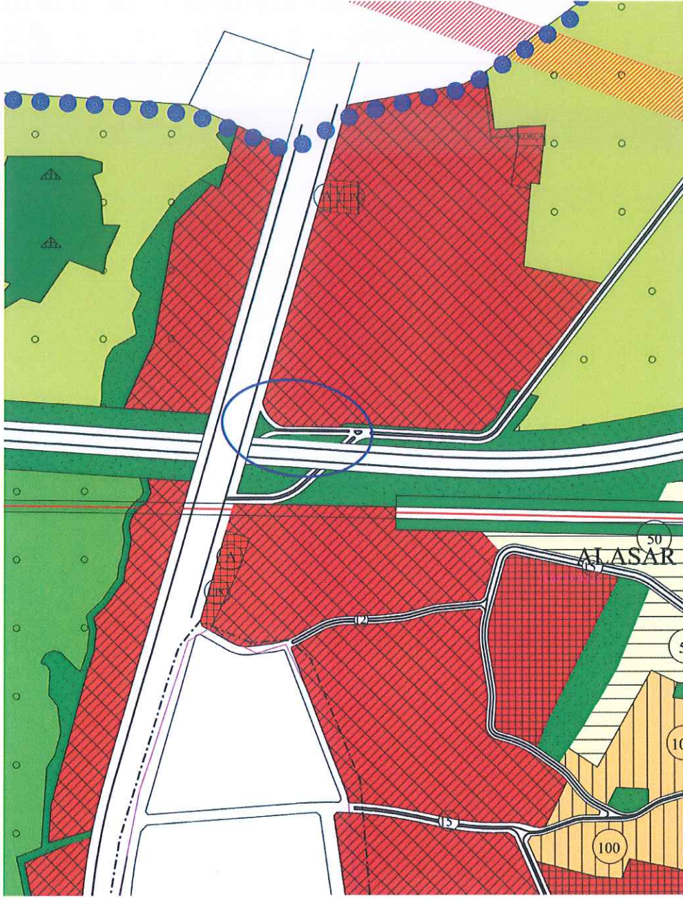
Onaylı 1/5000 ölçekli Nazım İmar Planı
