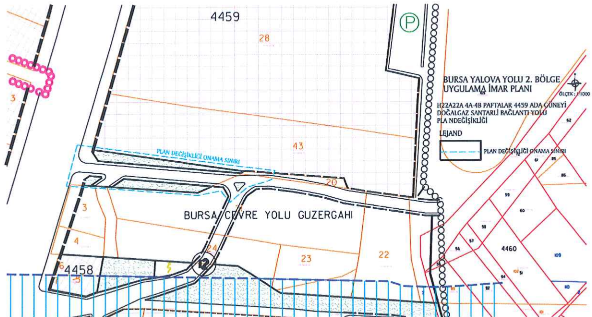
1/1000 ölçekli Plan Değişikliği önerisi
